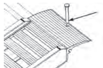
serienmäßige Bohrung in Auflagefläche für Abrutschsicherung mittels Bolzen
