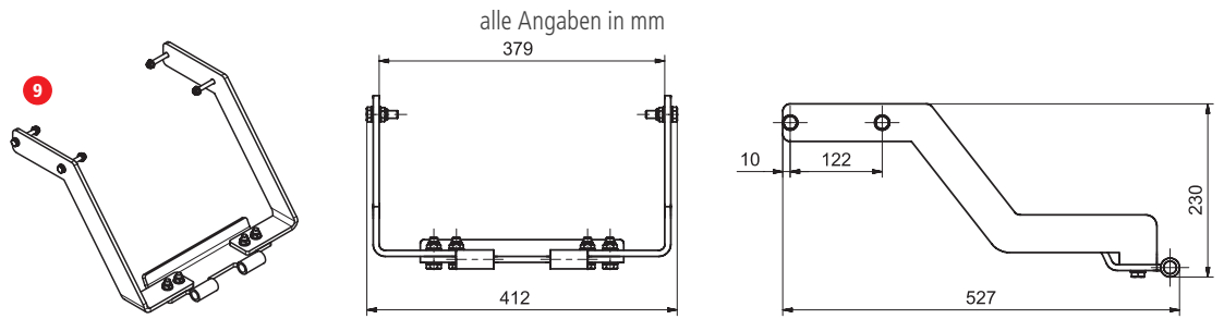
Adapter Viking, Stihl RT-Serie, AL-KO „Kleines Chassis“
