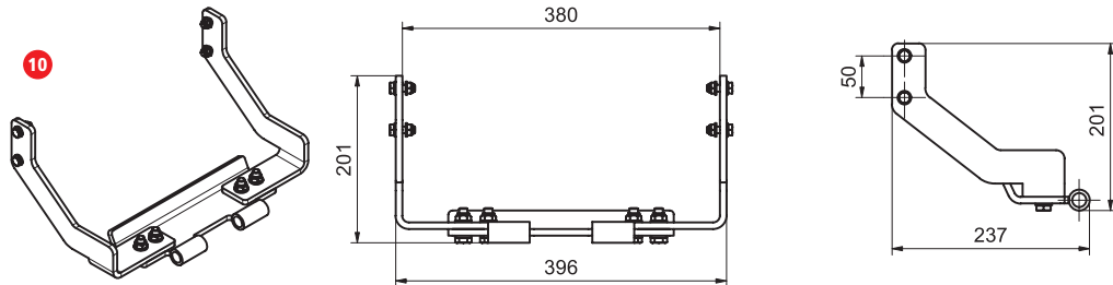
Adapter Viking, Stihl, AL-KO T-Serie
